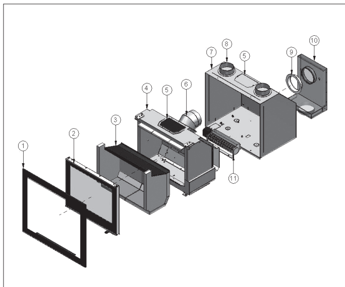
Linear inzethaard 600-900 (S,M,L,XL)
